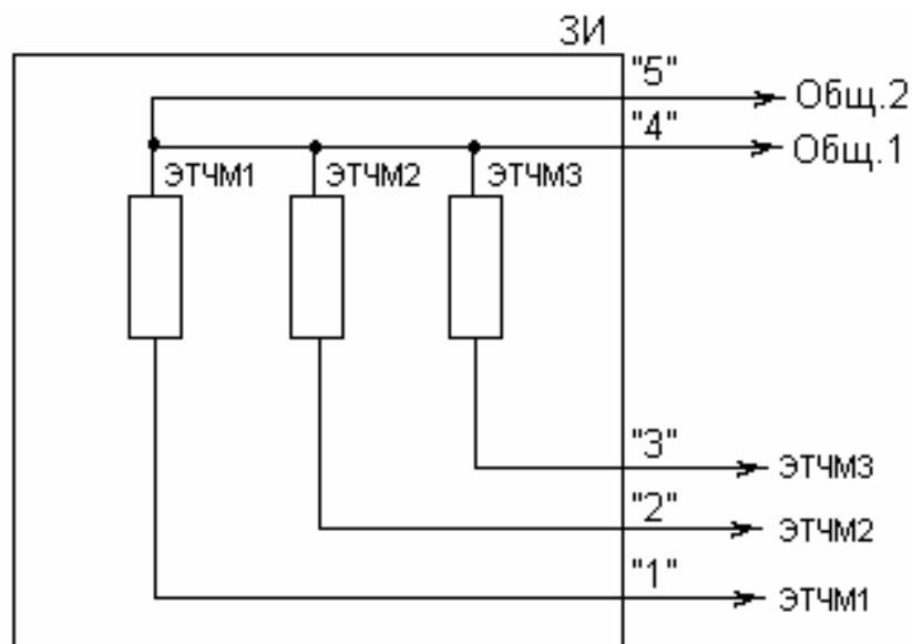
Рисунок 1.2 - Функциональная схема ЗИ
